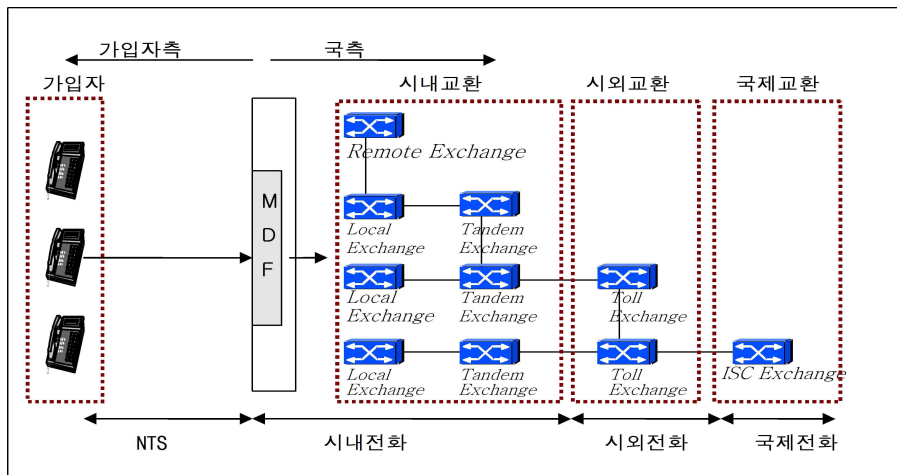
(그림 II - 1) 전화서비스 망 구성도
