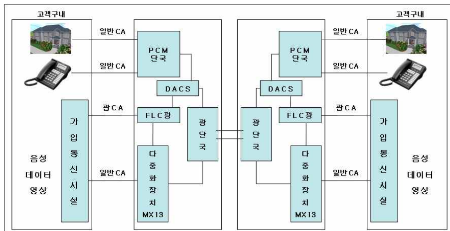
(그림 II - 5) 회선설비임대역무 망 구성도
