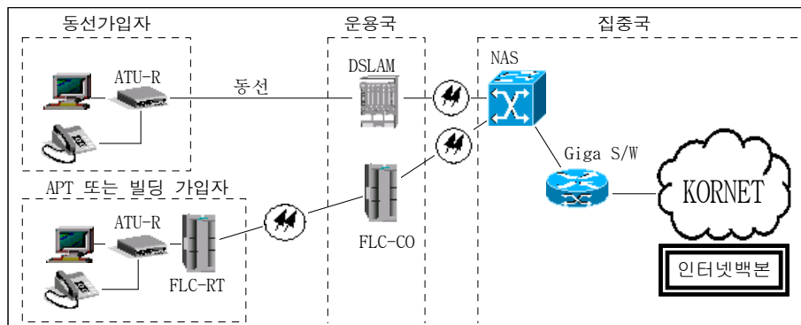
[그림 II-2] 인터넷가입자접속망 구성도
