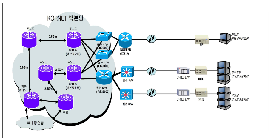
(그림 II - 3) 인터넷전용회선 망 구성도
